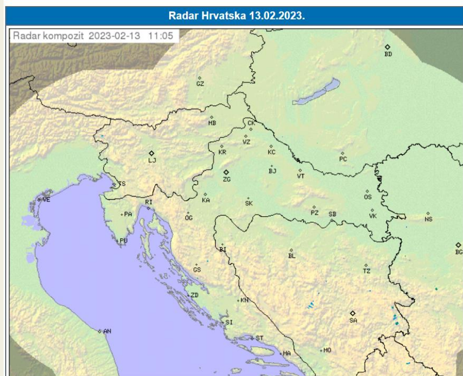
Radarska slika oborina - Hrvatska 13.02.2023.
