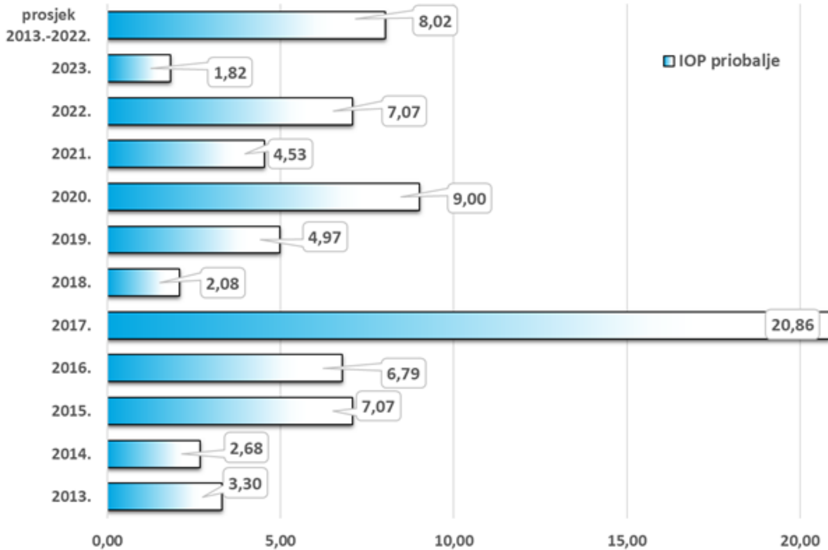
Indeks opožarene površine za priobalno i kraško područje 2013-2022. i 2023.
