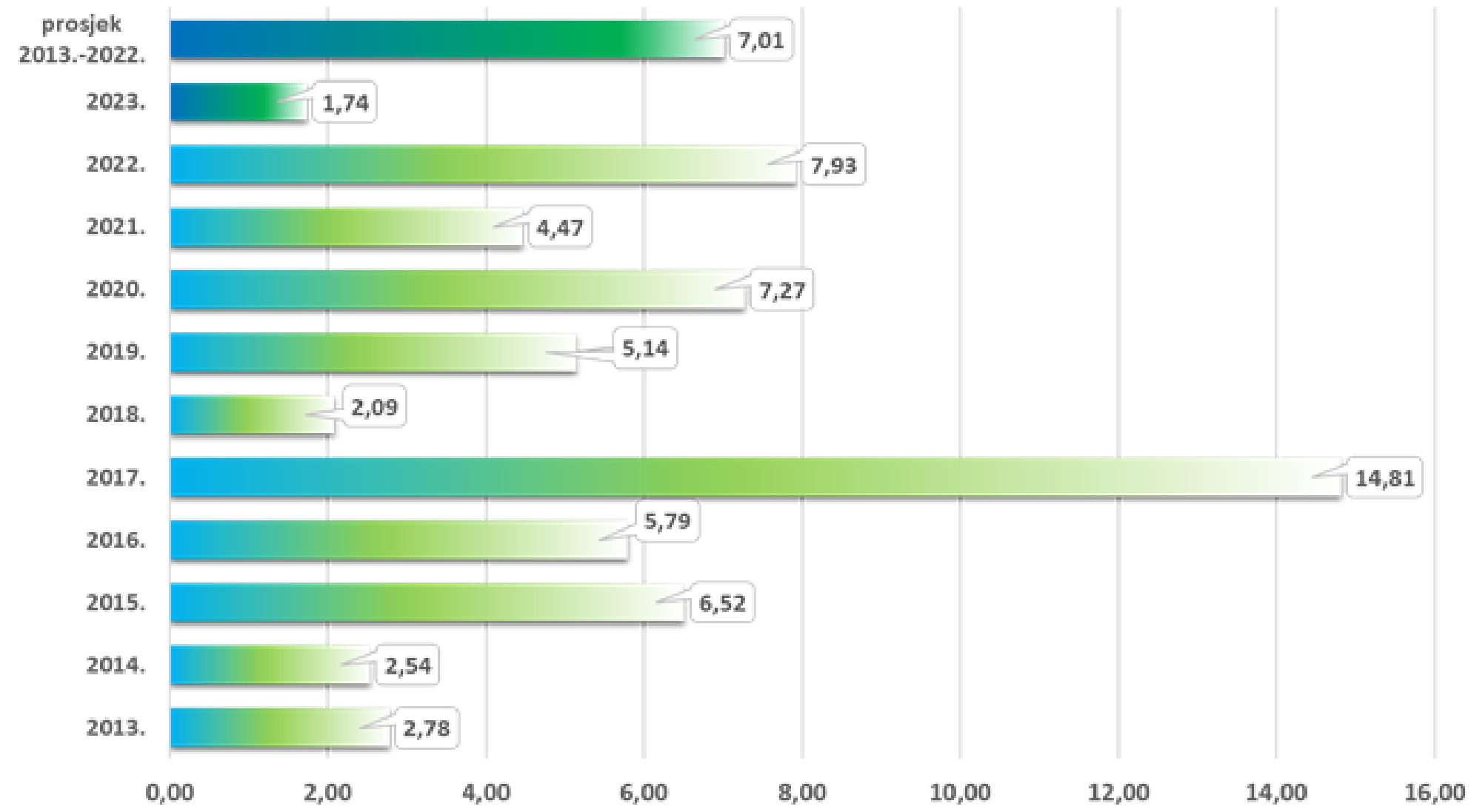
Indeks opožarene površine (IOP) za područje cijele RH
