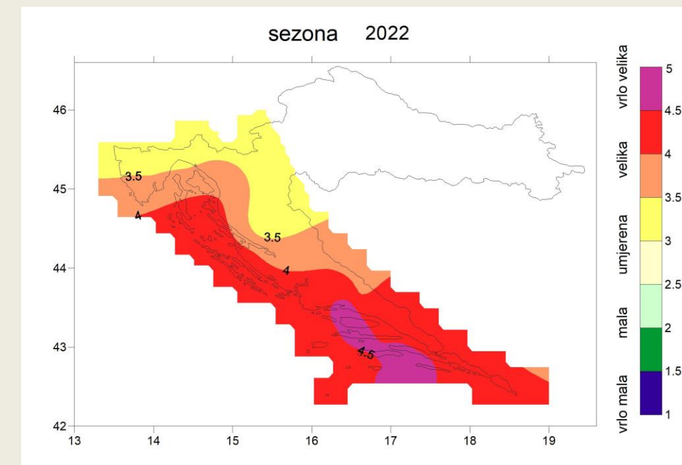
Slika 2.: Srednja mjesečna klasa opasnosti od požara raslinja za ljeto (lipanj, srpanj i kolovoz) 2022.
