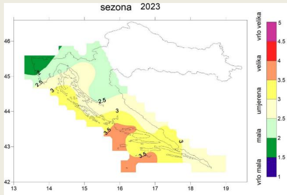
Slika 1.: Srednja mjesečna klasa opasnosti za nastanak i širenje požara raslinja za ljetnu sezonu (lipanj, srpanj i kolovoz) 2023.
